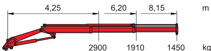
a2 8,28 m max. hydraulische Reichweite( Arm gestreckt) / max. outreach(horizontal position).
