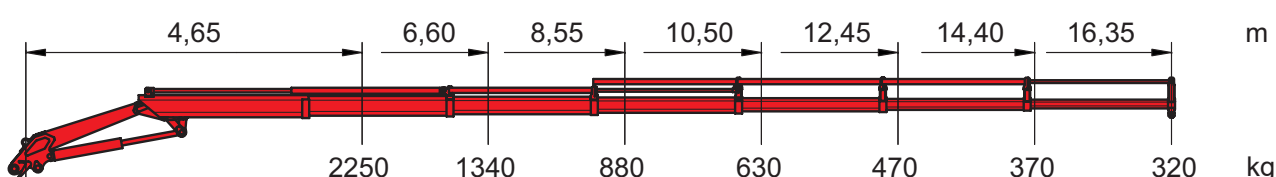
a6 16,48 m max. hydraulische Reichweite( Arm gestreckt) / max. outreach(horizontal position).
