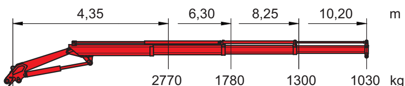
a3 10,33 m max. hydraulische Reichweite( Arm gestreckt) / max. outreach(horizontal position).
